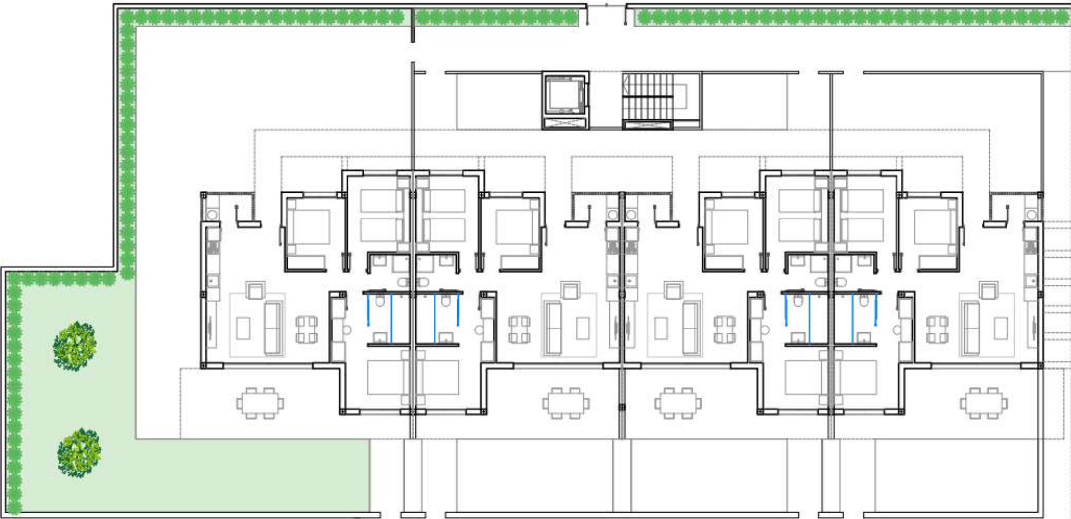
PLANTA BAJA
